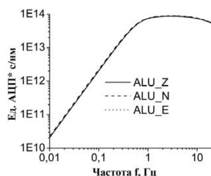
Рис. 3. Калибровочные кривые с/ст. «Алушта».
