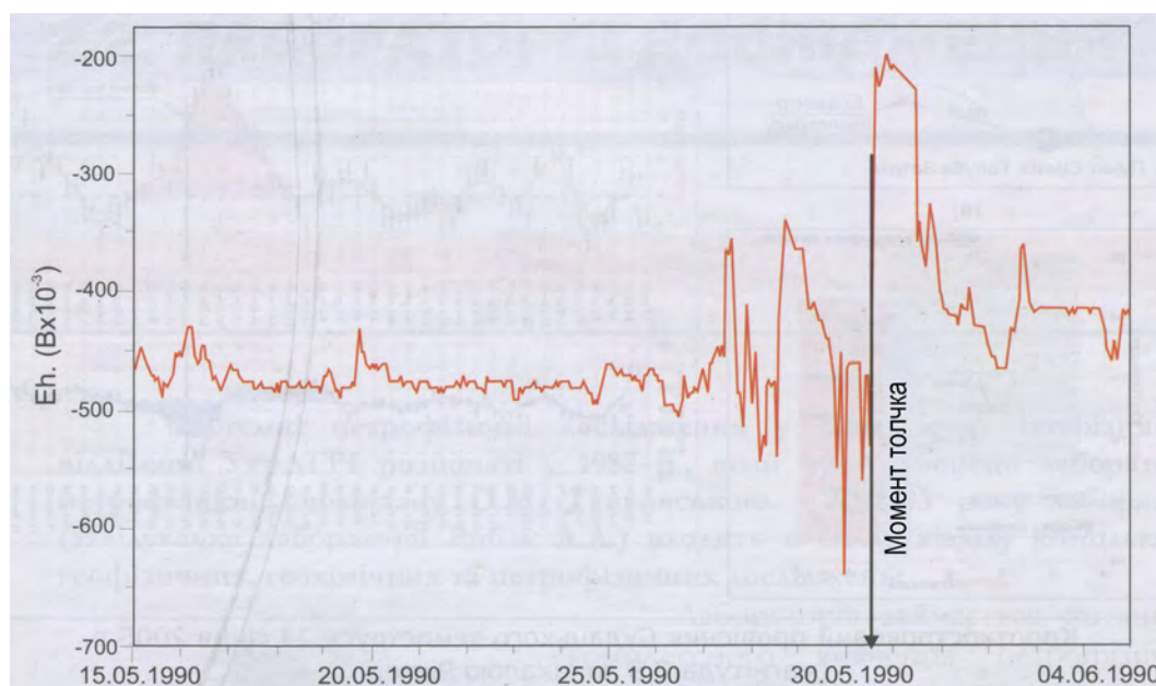
Рис. 2. Краткосрочный предвестник ЗТ 30.05.1990, произошедшего в зоне Вранча с магнитудой 7.1, зарегистрированный в вариациях окислительно-восстановительного потенциала Eh в пункте Красные Пещеры, скважина № 1 [6].
