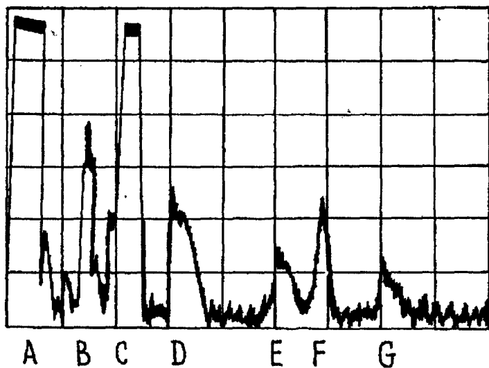
Рис. 3. Множественная структура сигнала эхо от ядер ^{53}\text{Cr} в \text{HgCr}_2\text{Se}_4 .
